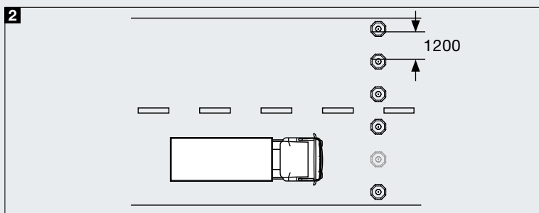
Avsperring i ubegrenset bredde med muligheten for å raskt og enkelt lage en passasje for autoriserte kjøretøy
