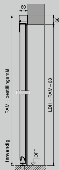
Sidedør med alu-blokkarm, profiltype 2 Montering bak åpningen
