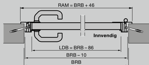
Sidedør med alu-hjørnekarm profiltype 3 Utvendig montering
