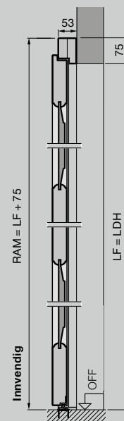
Sidedør i massivt tre Montering bak åpningen
