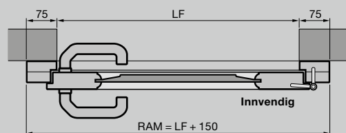
Sidedør i massivt tre Montering bak åpningen
